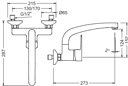
Grifo de cocina monomando mural 15 cm, caño largo Wall single-lever sink mixer 15 cm, long spout
