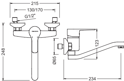
Grifo de cocina monomando caño inferior elevado K8 K8 Wall single lever sink mixer low spout
