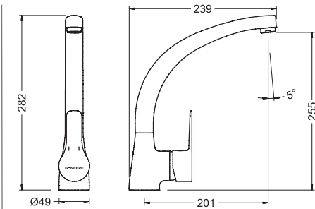
Grifo de cocina monomando caño conformado K8 K8 Single-lever sink mixer tube spout
